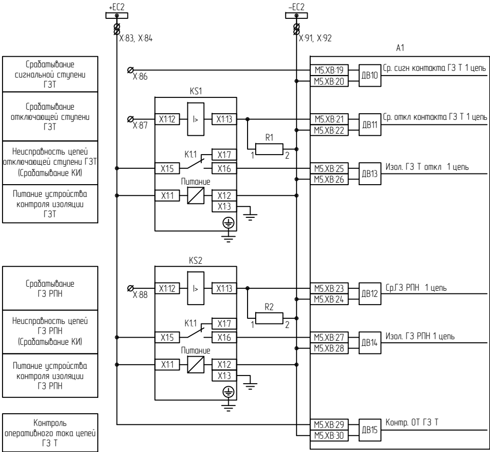
Цепи оперативного тока ГЗ Т А1
